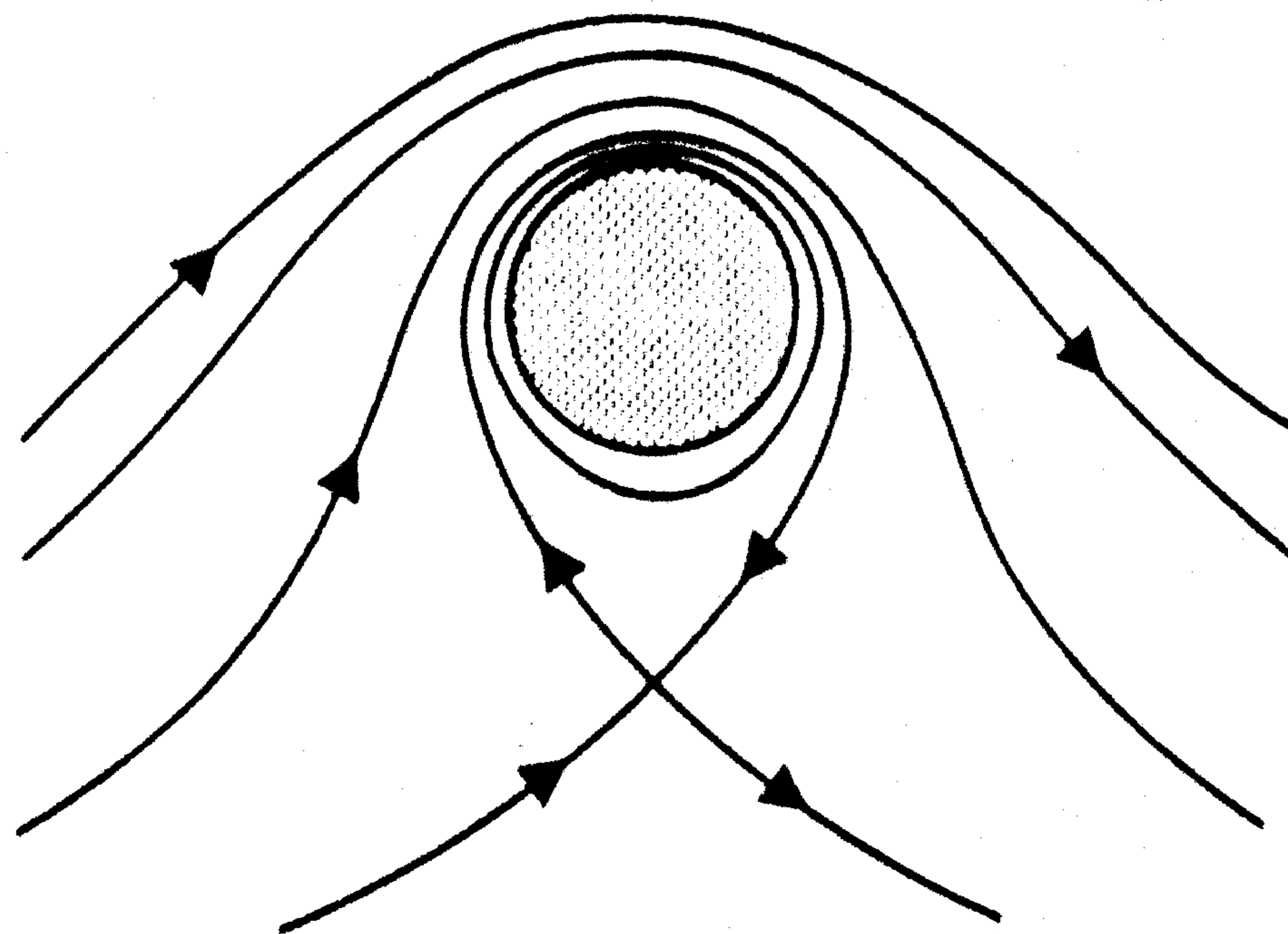
(d) B > 2
