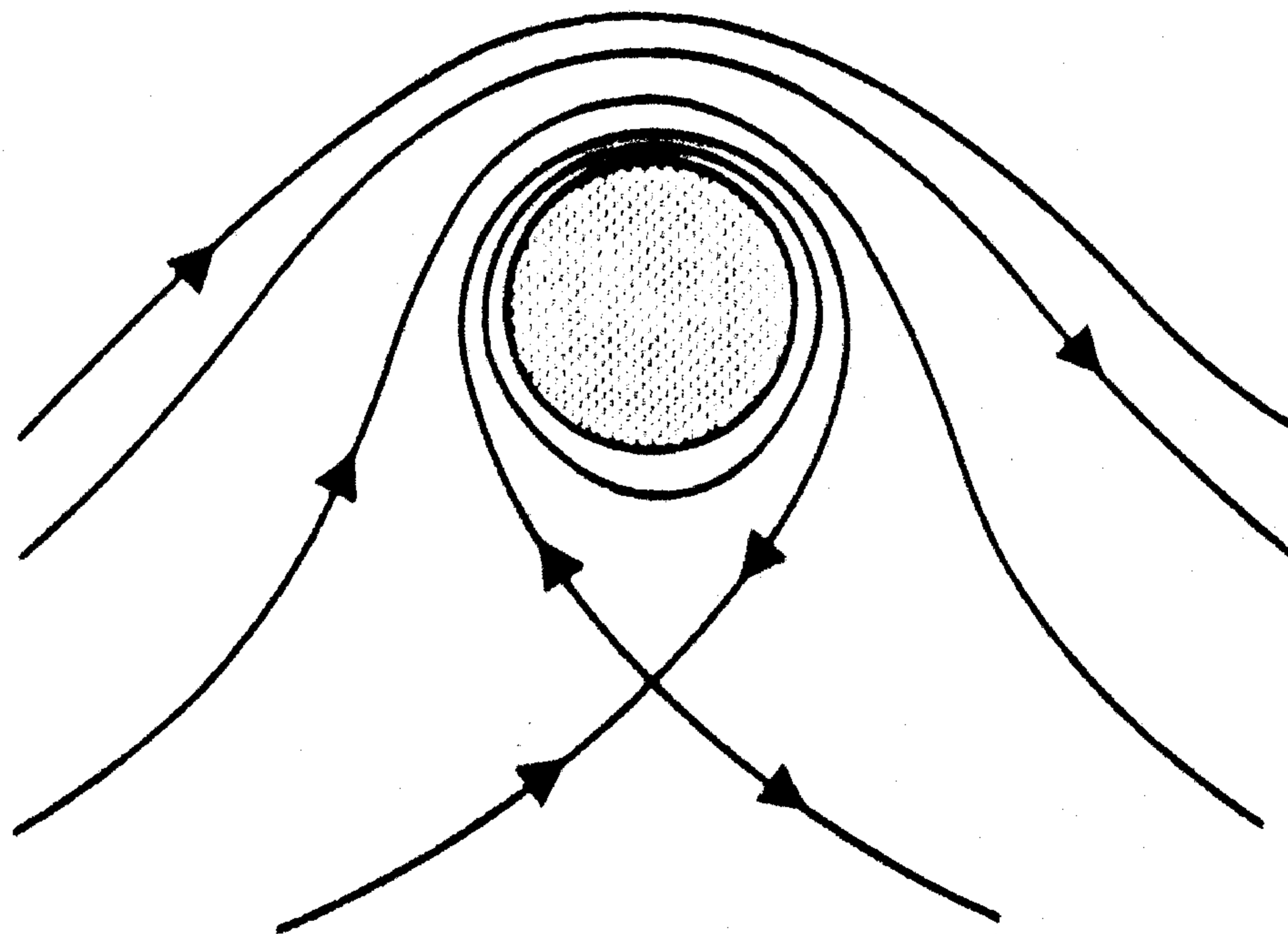
(d) B > 2
