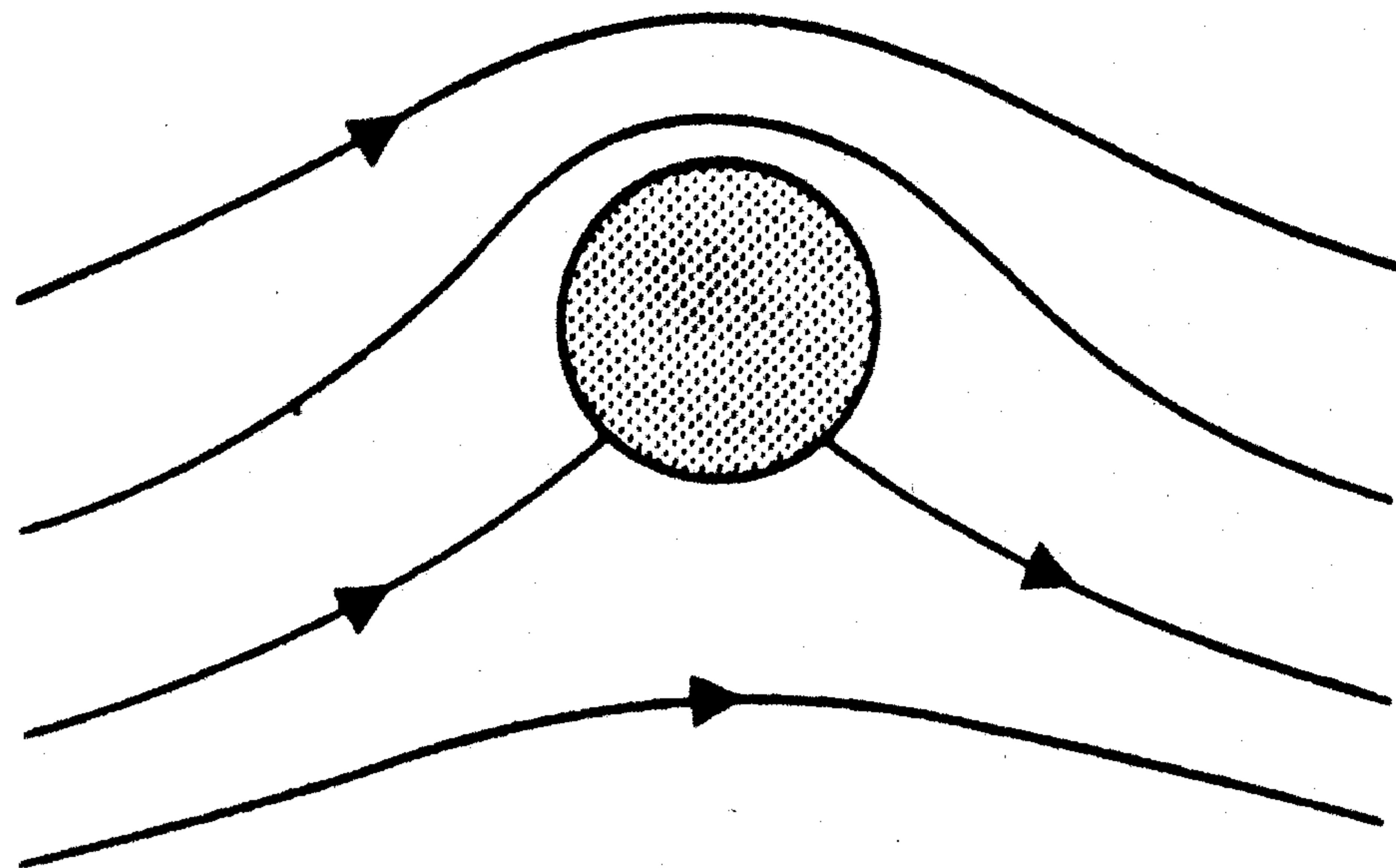
(b) B < 2
