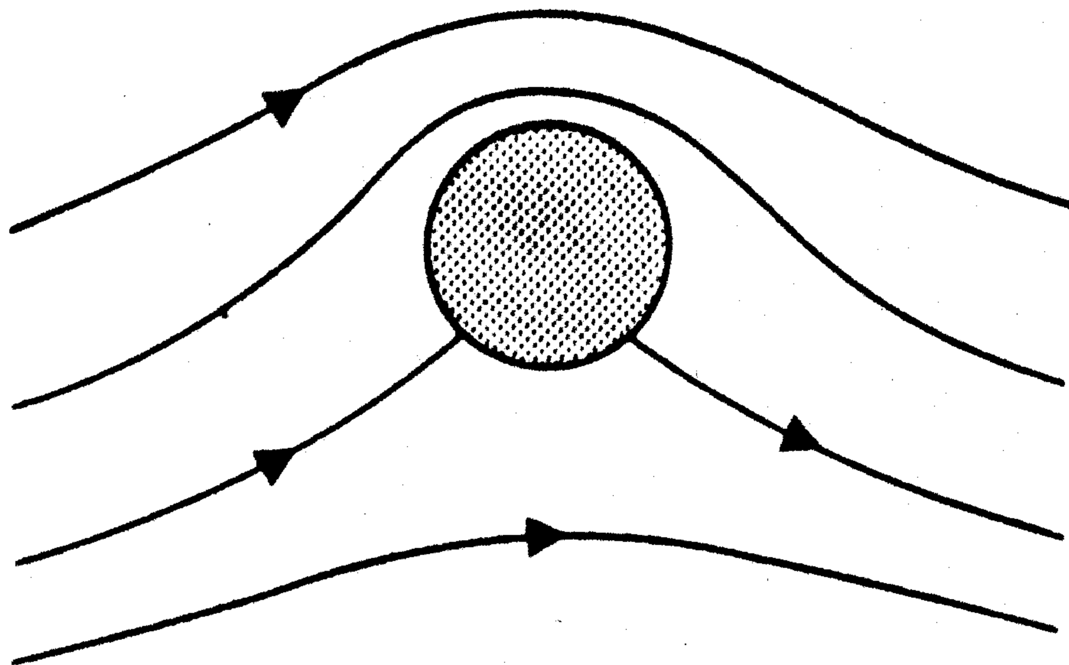
(b) B < 2
